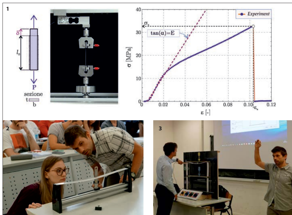
1. Dalla prova di laboratorio alle costanti elastiche. / From the experimental test to the elastic moduli. 2,3. Dal calcolo teorico alla verifica sperimentale dei risultati attesi. / From the theoretical results to their experimental validation.
