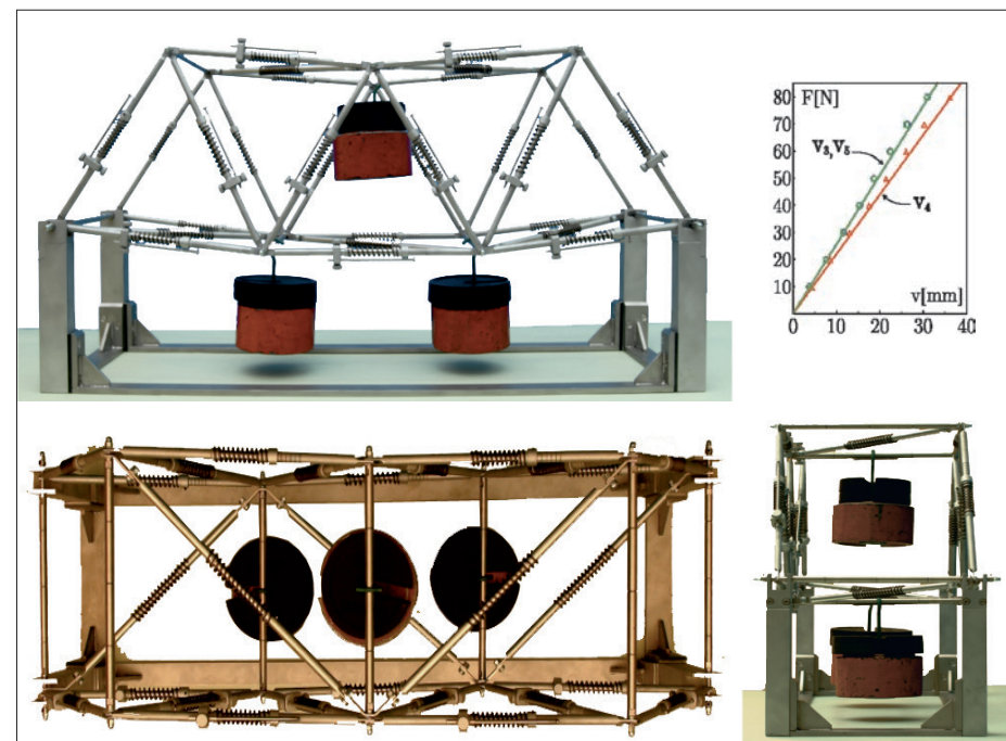
Calcolo di strutture reticolari e verifica sperimentale dei risultati / Structural analysis of truss structures and experimental proof of the theoretical predictions
